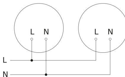
Schema elettrico Master-Master Bluetooth collegamento in rete
